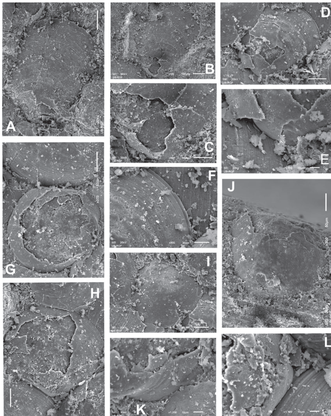
Slika 3 (A-L). Detaljne SEM fotografije ljušturica školjaka iz Plaskovačke formacije pokazuju razlike u obliku, veličini i morfometriji ljuštura (broj kod svakog primerka prikazuje maksimalnu dužinu ljuštura u µm). Detaljne SEM fotografije juvenilne faze rasta za primerke: A, B (C je detalj od slike B i pokazuje prodizoknh). Slika 3 (D-L)-detaljne SEM fotografije rane postlarvalne faze za primerke: D, E (E-detalj od sl. D, pokazuje prodizoknh), F (F-detalj od slike D, pokazuje ivicu kapka); G, K (K-detalj od slike G); H, L (L-detalj od H), slika pokazuje fragmente od dva primerka, na levom primerku se vidi gladak prodizoknh, a na drugom obod kapka sa komarginalnim linijama rasta (desni ugao slike).
