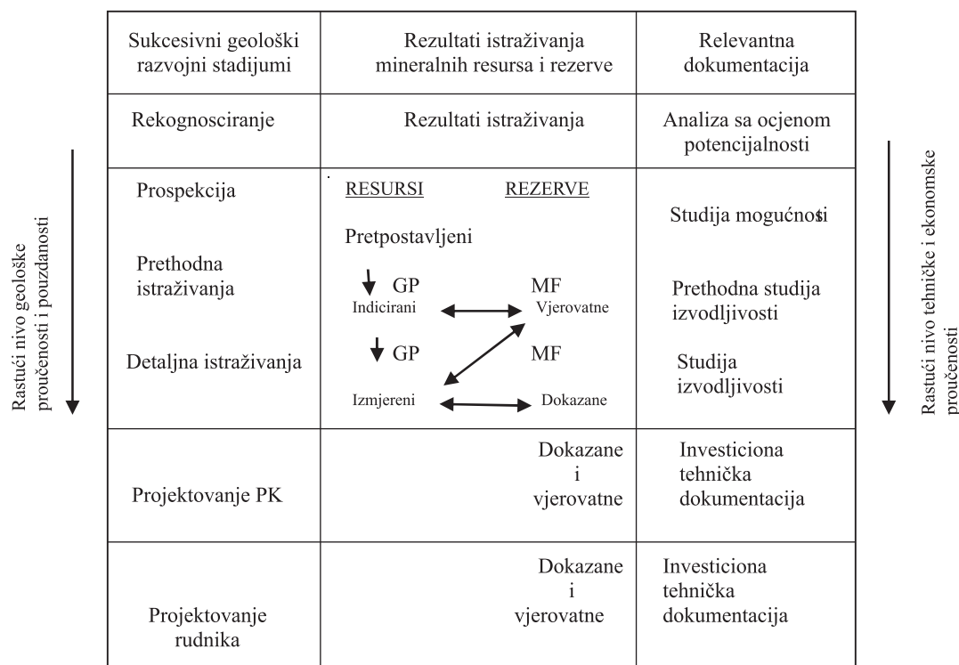
Slika 1. Opšti odnos između rezultata istraživanja, mineralnih resursa i mineralnih rezervi
