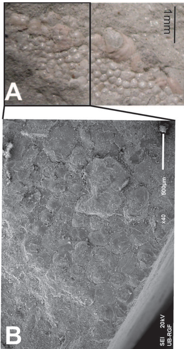
Slika 2 (A, B). Mikrofotografije grupnih ljušturica Dreissenidae iz Plaskovačke formacije (centralna Srbija).
